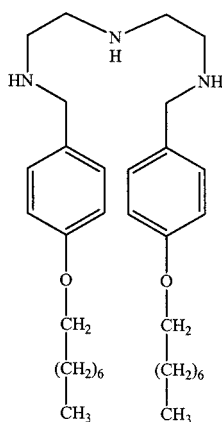
2,2'-bis( p -octyloxybenzyl)diethylenetriamine (bis- p ODET)
